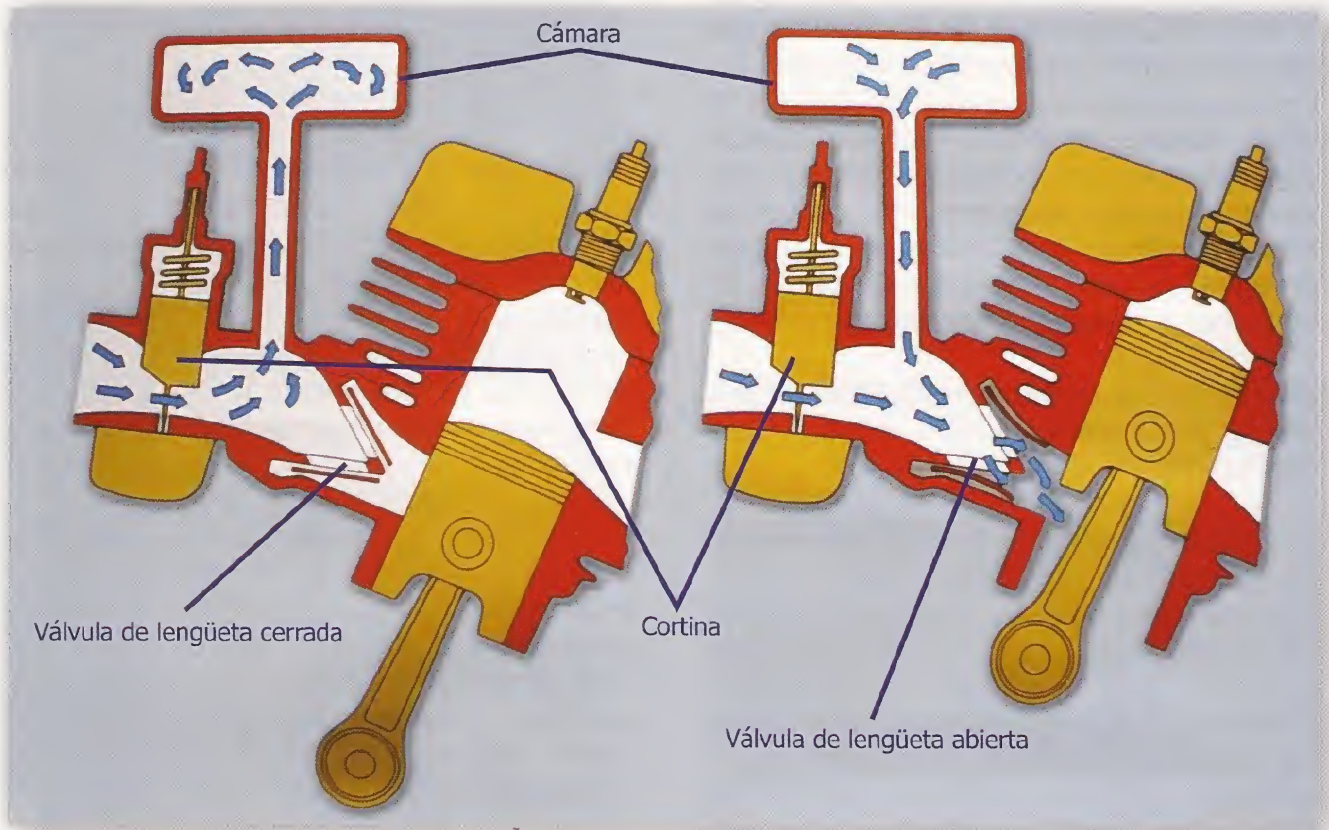
Diagrama de trabajo del sistema YEIS
